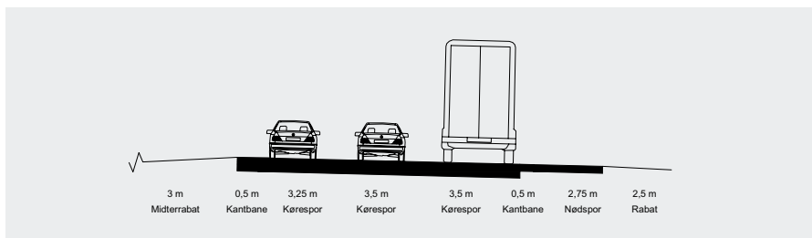
Figur 2.8 Normaltværprofil for udvidelse af motorvejen til 3 spor i hver retning.
