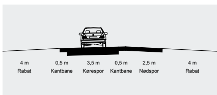
Figur 2.7 Normaltværprofil for til- og frakørsler i det nye tilslutningsanlæg.
