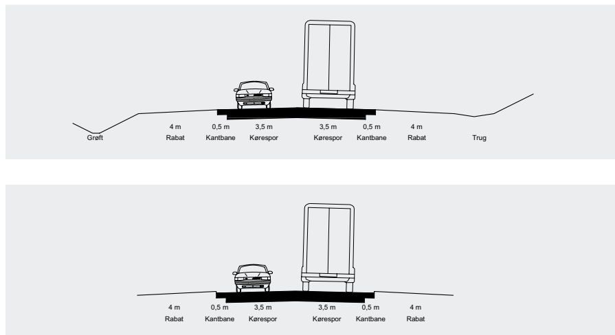
Figur 2.2 Normaltværprofil for Egnspanvej i hhv. påfyldning og afgravning samt ved kantopsamling.
