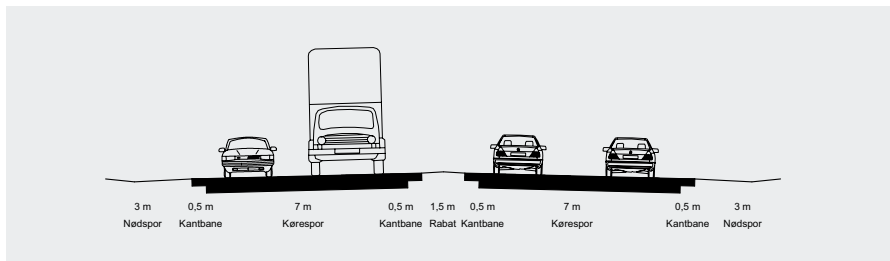
Figur 2.5 Normaltværprofil for motorvejsbroen der forbinder de to rampekryds.
