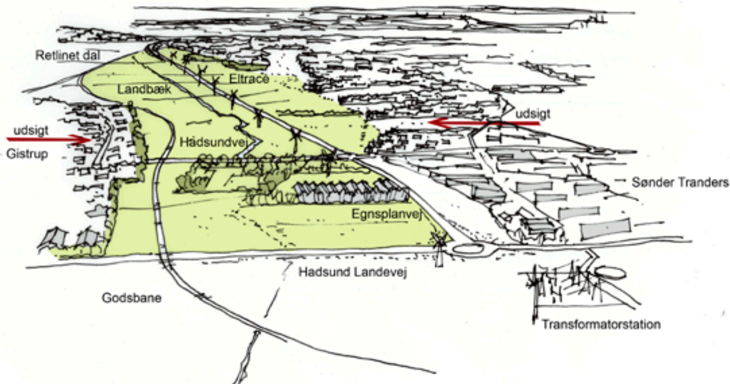
Figur 4.3 Vejtracé fra Hadsund Landevej til tilslutning med Zeusvej. Vejtracéet løber gennem åbent land midt i Indkilledalen (St.5478-st. 2475).
