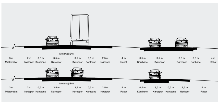
Figur 2.6 Normaltværprofiler for parallelsportene, med og uden sportilføjelse.
