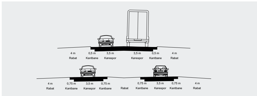
Figur 2.10 Normaltværprofil for Ny Dallvej og for delstrækningen, hvor de to kørespor forløber i delt tracé.
