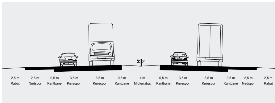
Figur 2.12 Normaltværsprofil for motorvejsindføringen til City Syd.
